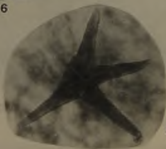
Fig. 1. Drimys winteri , estoma cara abaxial, 850x; SGOpm. 885. Fig. 2. Laurelia sempervirens , estomas cara abaxial, 300x; SGOpm. 878. Figs. 3-6. Laureliopsis philippiana , cara abaxial, 3. estomas, 500x; 4. pelo simple, 320x; 5. escama, 500x; 6. tricoma malpighiáceo, 225x; SGOpm. 511. Figs. 7-8. Peumus boldus , cara abaxial, 7. estoma, 350x; 8. pelo estrelado, 140x; SGOpm. 738.
