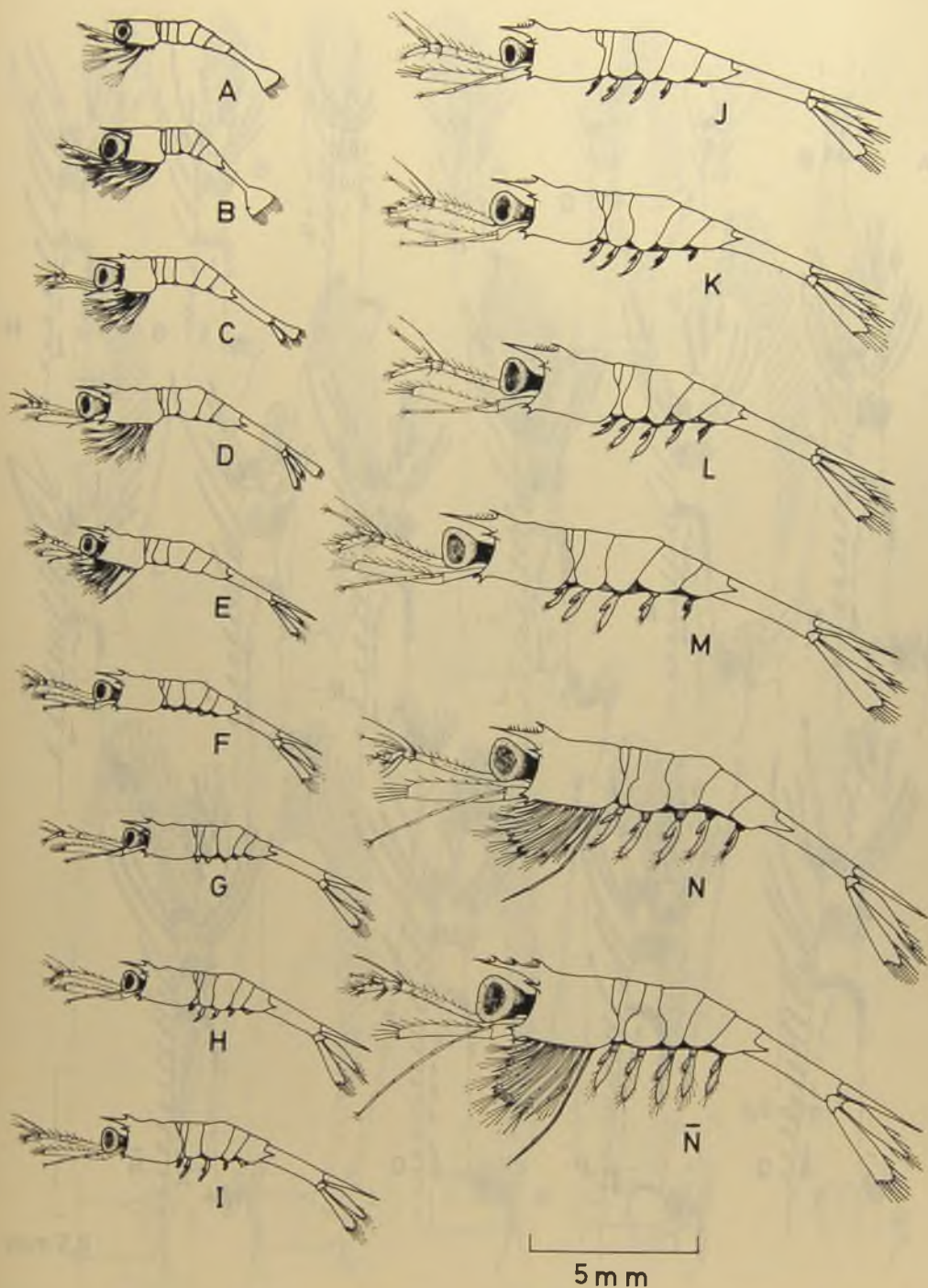
Fig. 1 Estadios misis del desarrollo larvario de Cryphiops caementarius : A, I; B, II; C, III; D, IV; E, V-VIII; F, IX; G, X; H, XI; I, XII; J, XIII; K, XIV; L, XV; M, XVI; N, XVII; Ñ, Post misis (megalopa).
