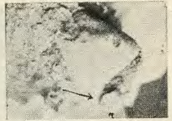
Fig. 2.—CARDITA sp. 3/4 Corral de Barrancas. Fossilifero N.º 4. b) 1/1. Molde interno mostrando la impresión muscular
