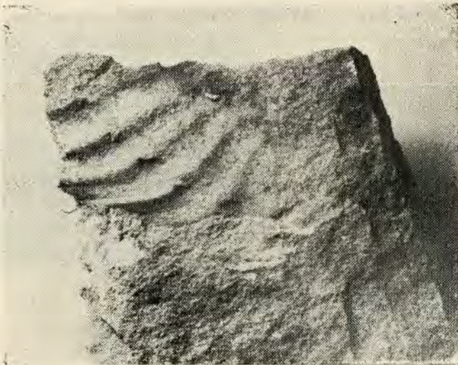
Fig. 2.—Amonite. 1/1. Los Placeres. Punto Fosilifero N.º 6.
